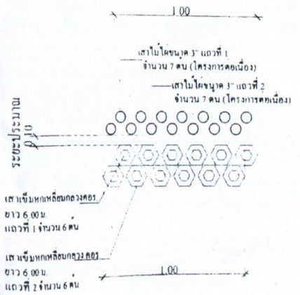
ขยายการปักเสาป้องกันน้ำกัดเซาะตลิ่ง SCALE
